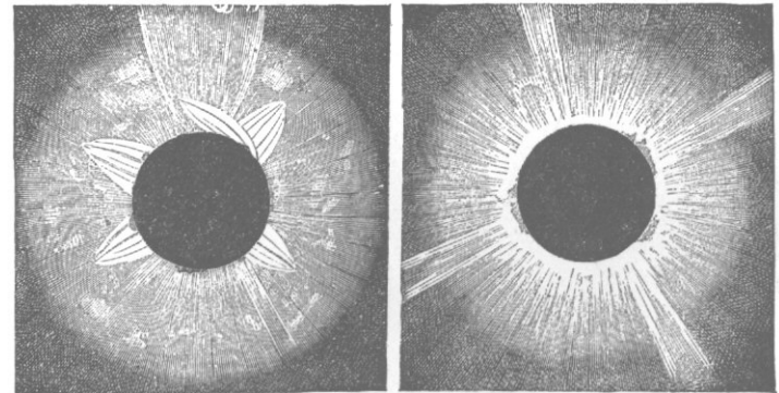
Fig. 154. Eclipse of 1858 (Liais).
