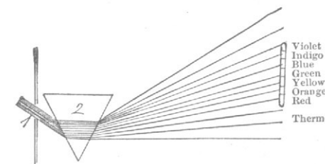
Fig. 173. The Spectrum.
