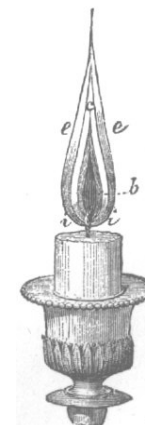
Fig. 162.
